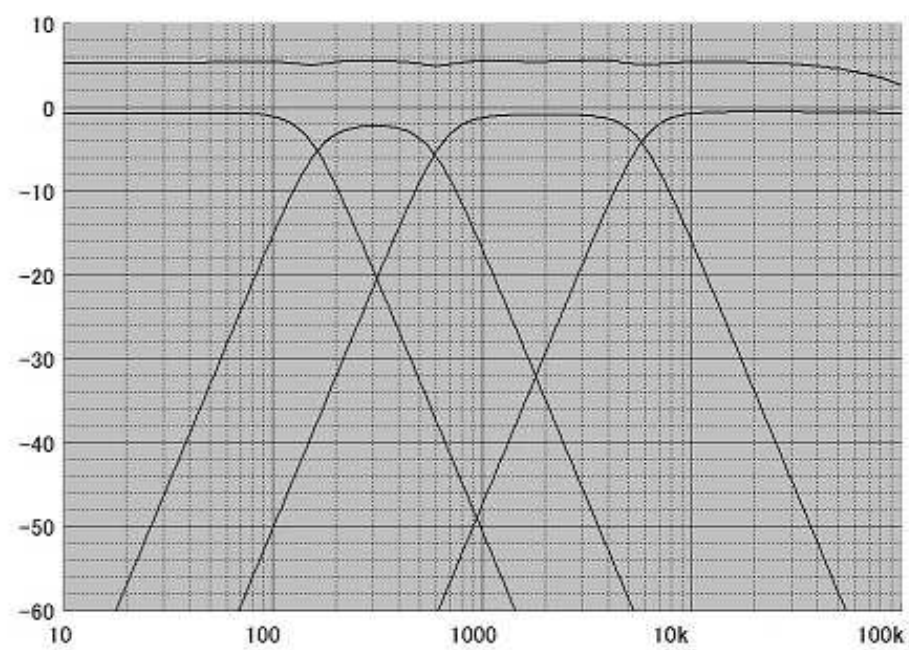
18dB/octバターワース補正後
