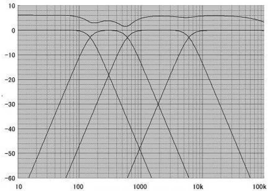
18dB/octバターワース補正前
