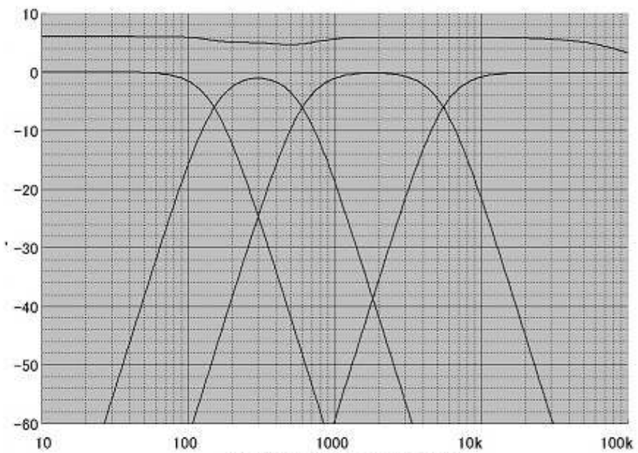
24dB/octリンクウイツ補正前
