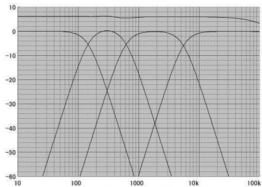
24dB/octリンクウイツ補正後
